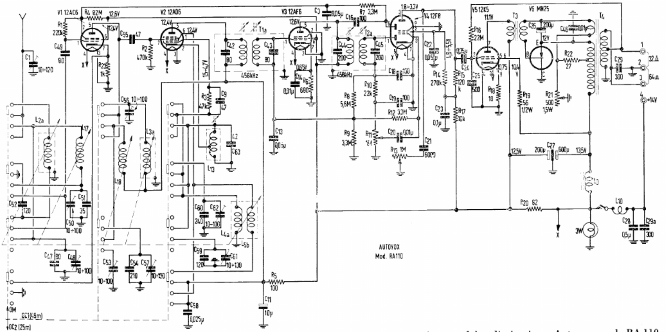
Schema elettrico del radioricevitore Autovox, mod. RA 110
